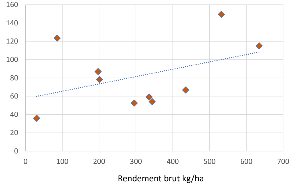
Indice de Shannon Macro-Invertébrés
